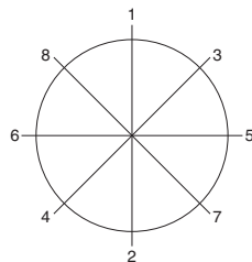
図14-B (8本ボルト)
