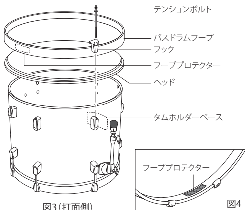
図3 (打面側)
